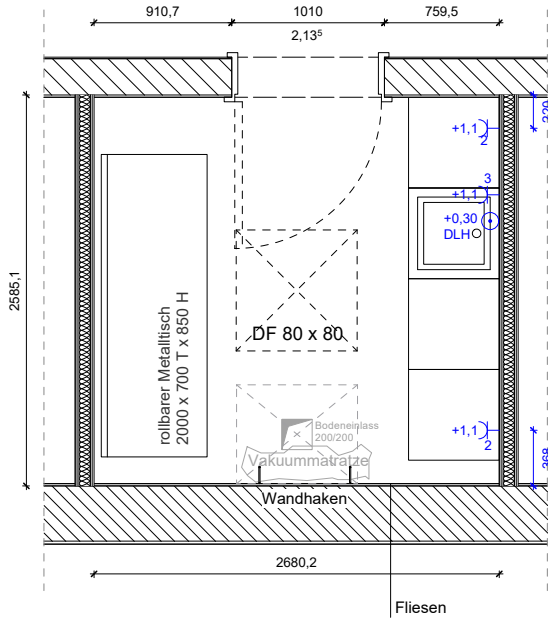
Grundriss Desinfektion 1:50
