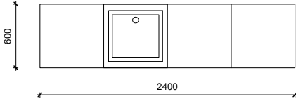
00.17.02 - 05 Draufsicht Spülbecken:
