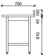
Queransichten:
