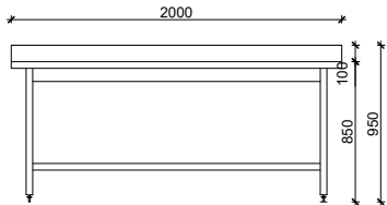
00.17.01 Rollbarer Metalltisch Längsansicht:
