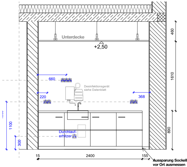
Ansicht Desinfektion 1:50
