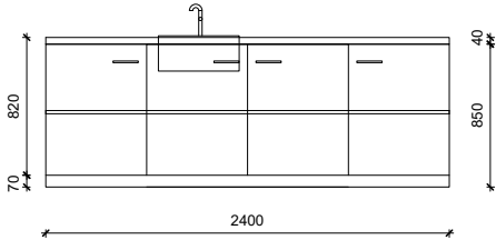
Längsansicht:
